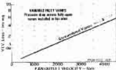
Fig. 3 V.I.V. Losses
